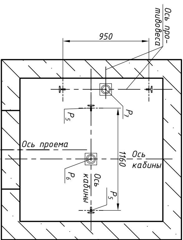
План прямка В-В
