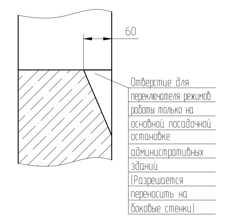
К-К (1:5) (2,4)
