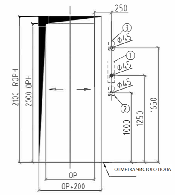
ЭТАЖИ
