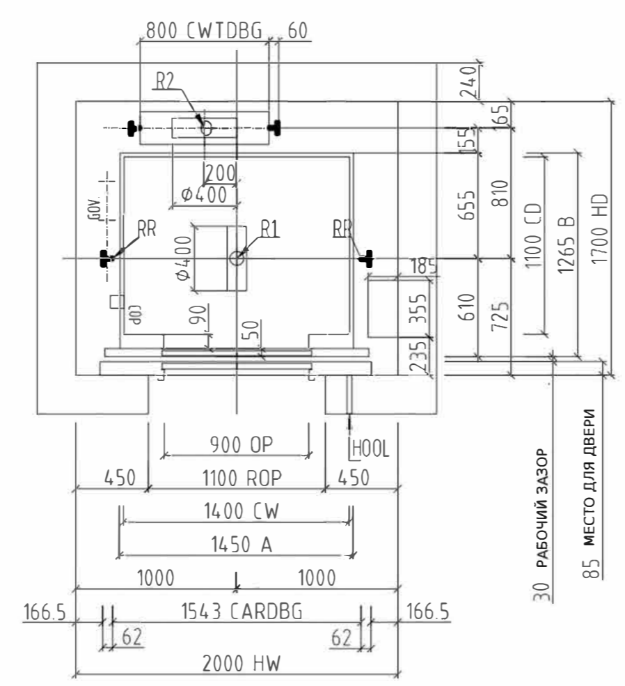
ПЛАН ШАХТЫ
