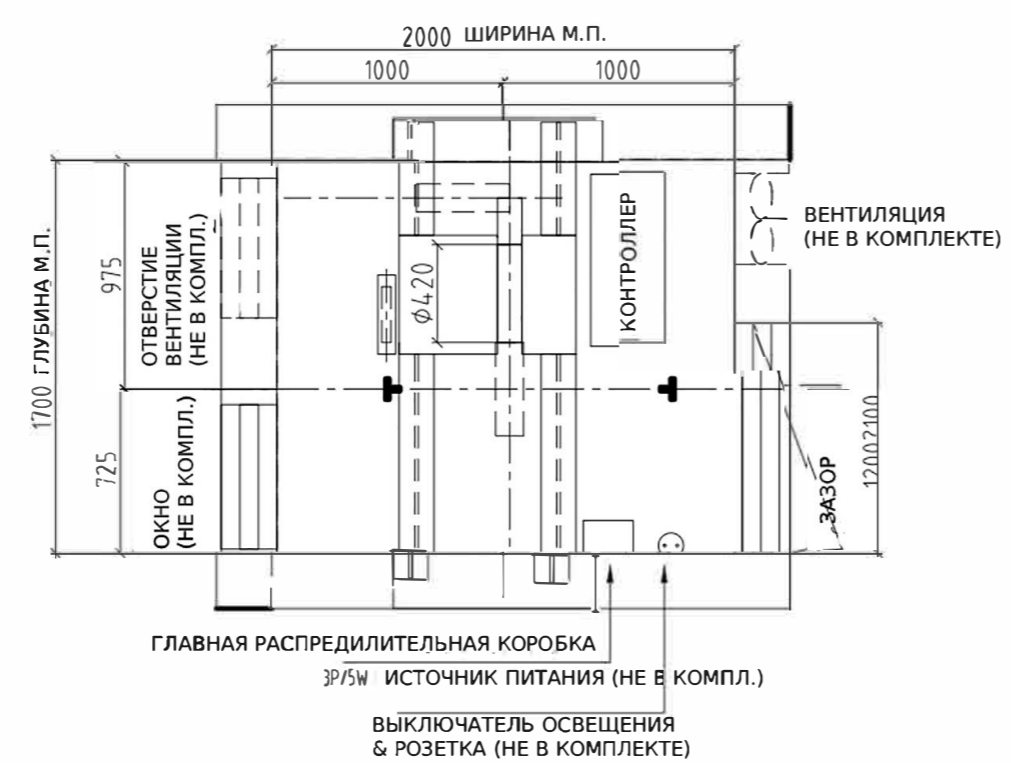
МАШИНОЕ ПОМЕЩЕНИЕ
