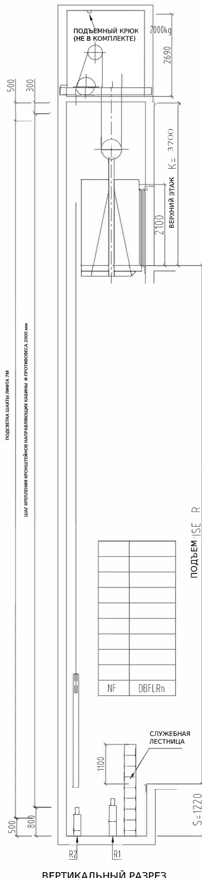
ВЕРТИКАЛЬНЫЙ РАЗРЕЗ
