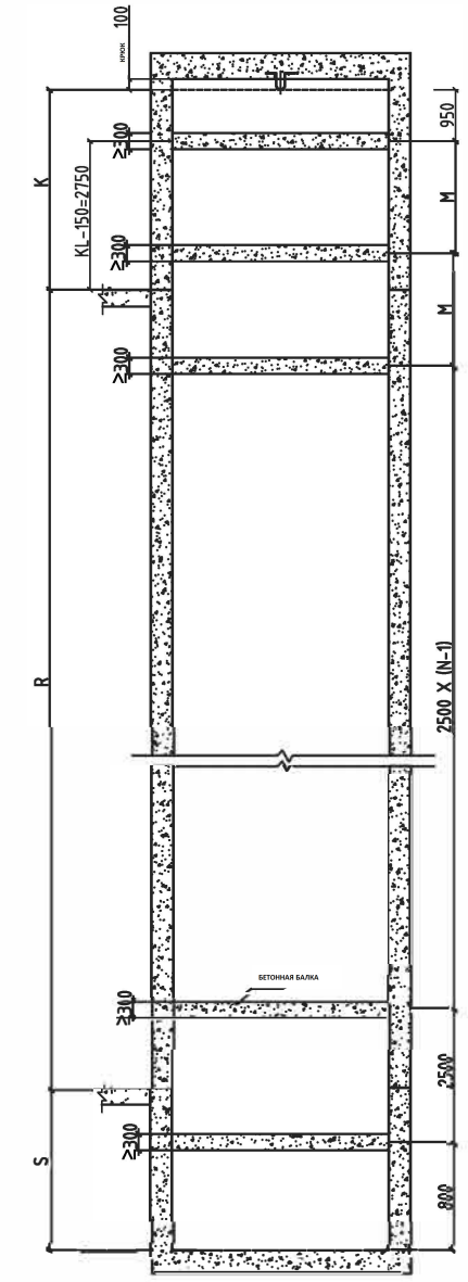
ЛЕВЫЕ БЕТОННЫЕ БАЛКИ (ВИД: ЛИЦОМ К ДВЕРИ)
