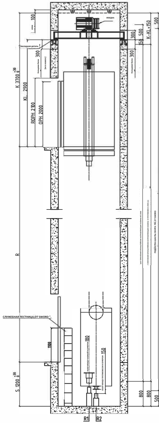
ВЕРТИКАЛЬНЫЙ РАЗРЕЗ
