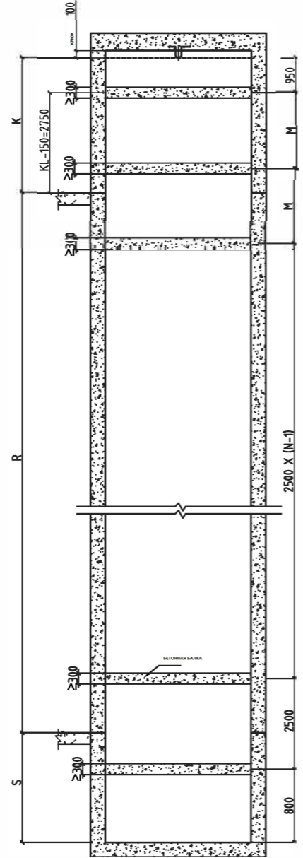
ЛЕВЫЕ БЕТОННЫЕ БАЛКИ (ВИД: ЛИЦОМ К ДВЕРИ)
