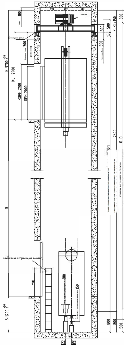
ВЕРТИКАЛЬНЫЙ РАЗРЕЗ
