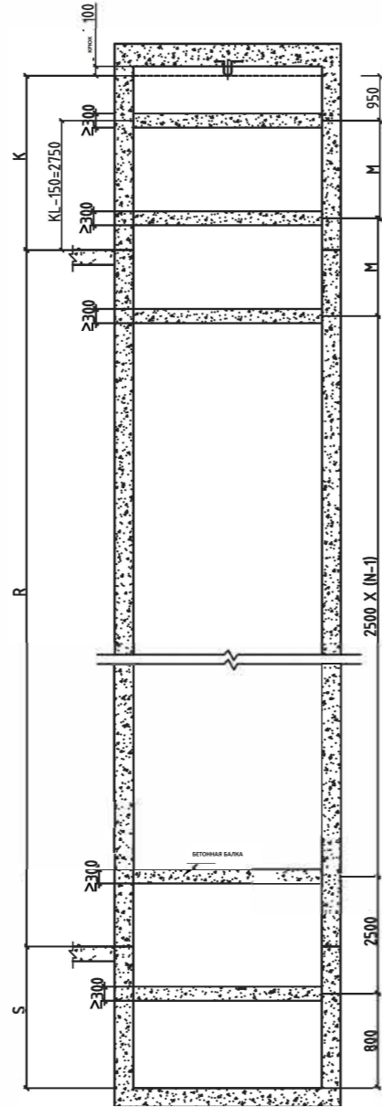
ЛЕВЫЕ БЕТОННЫЕ БАЛКИ (ВИД: ЛИЦОМ К ДВЕРИ)
