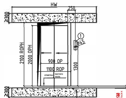
(ОСТАЛЬНЫЕ ЭТАЖИ)
