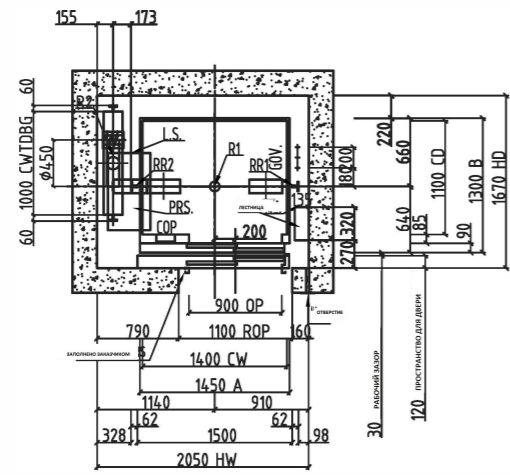
ПЛАН ШАХТЫ
