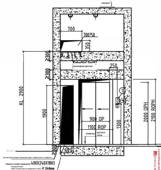
(ВЕРХНИЙ ЭТАЖ)
