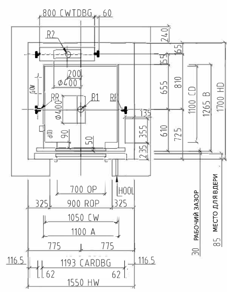
ПЛАН ШАХТЫ
