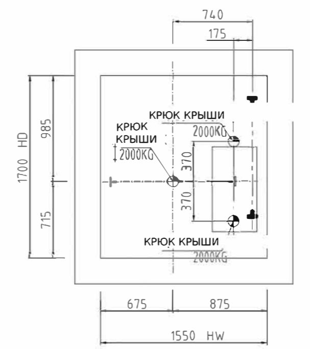
ПЛАН КРЮКА ВЕРХА ШАХТЫ (НЕ В КОМПЛЕКТЕ)
