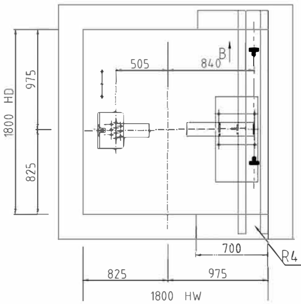
ПЛАН ВЕРХА ШАХТЫ
