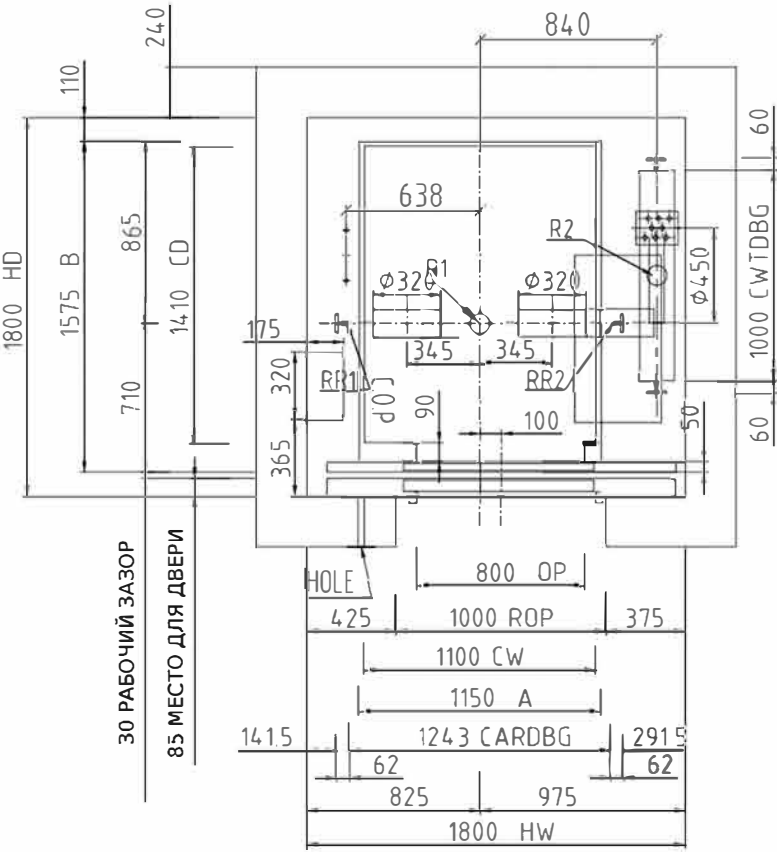
ПЛАН ШАХТЫ
