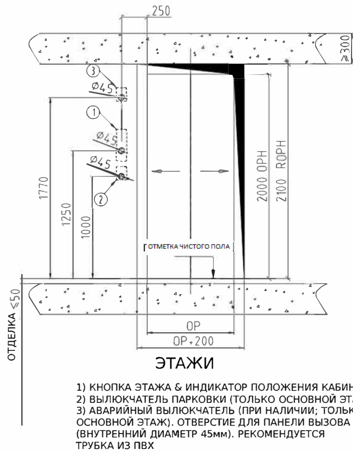
ВИД СПЕРЕДИ
