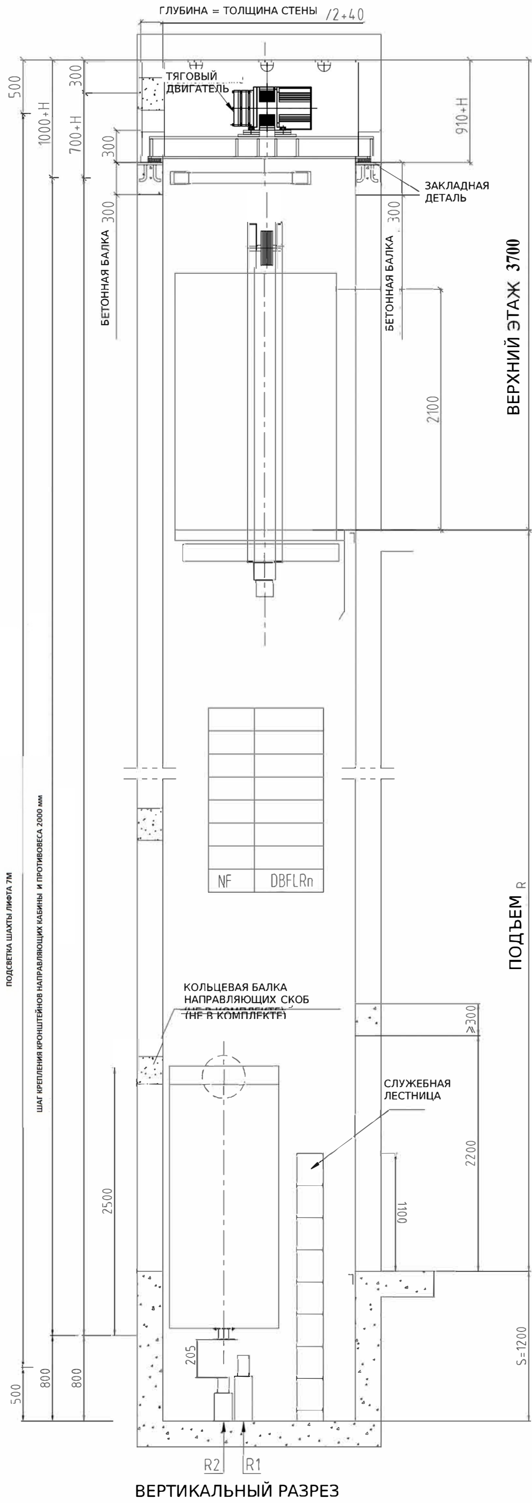
ВЕРТИКАЛЬНЫЙ РАЗРЕЗ
