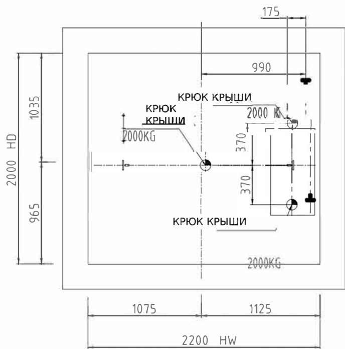
ПЛАН КРЮКА ВЕРХА ШАХТЫ (НЕ В КОМПЛЕКТЕ)
