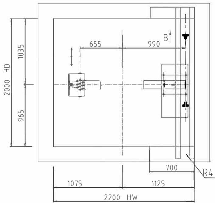
ПЛАН ВЕРХА ШАХТЫ
